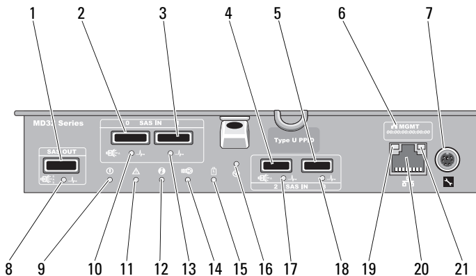
图 3-1. MD3200 系列 SAS RAID 控制器模块
