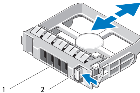
图 15-2. 卸下和安装 3.5 英寸硬盘驱动器挡片（仅限 MD3200）
