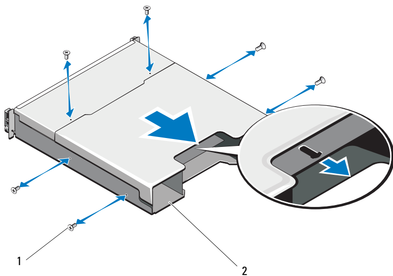
图 15-15. 卸下和安装 RAID 控制器模块 / 电源设备框架
