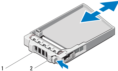
图 15-3. 卸下和安装 2.5 英寸硬盘驱动器挡片（仅限 MD3220）
