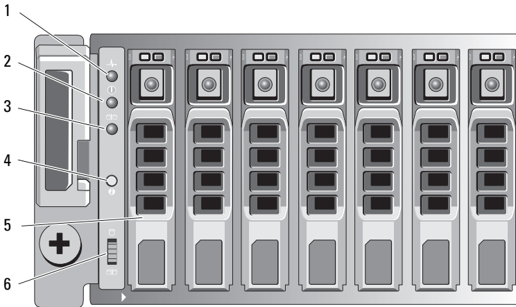
图 2-2. 前面板部件和指示灯 — Dell PowerVault MD3220
