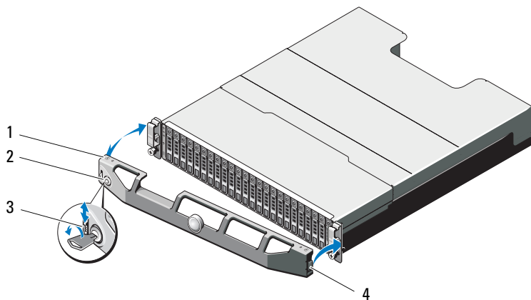
图 15-1. 卸下和安装前挡板
