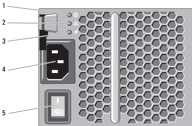
图 2-6. 电源指示灯代码和功能
