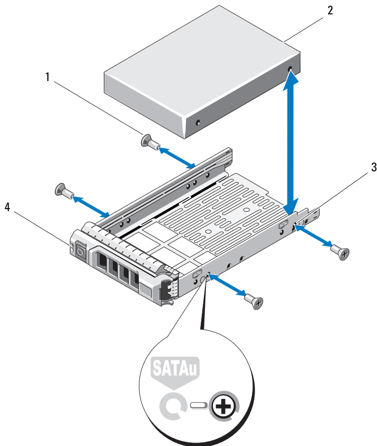
图 15-5. 卸除并安装硬盘驱动器到 3.5 英寸硬盘驱动器托盘中
