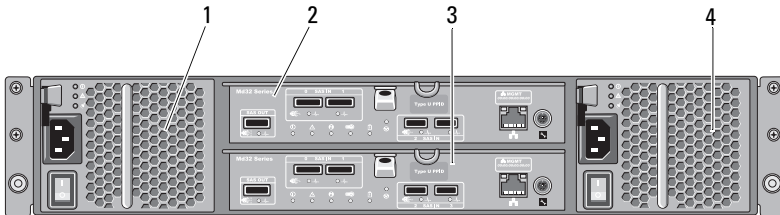
图 2-4. 背面板部件和指示灯—Dell PowerVault MD3200 系列
