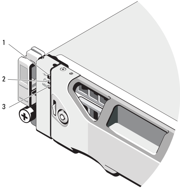
图 2-3. 前挡板部件和指示灯
