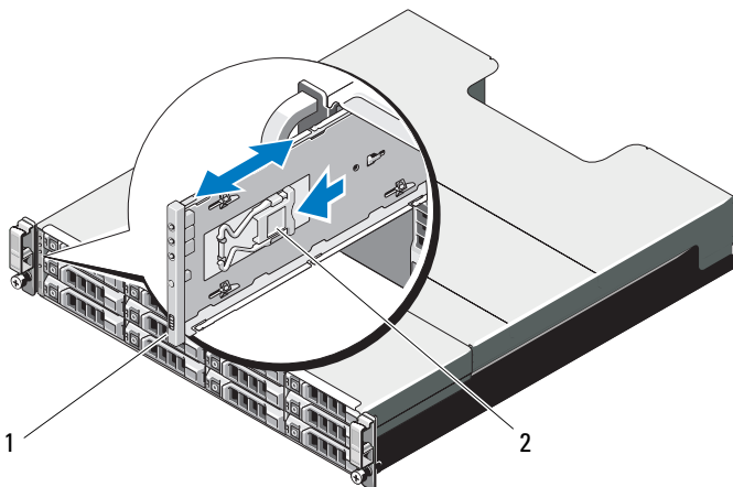
图 15-13. 卸下和安装控制面板 -PowerVault MD3200
