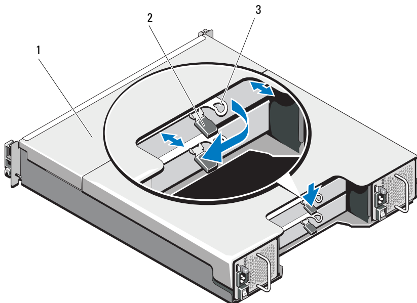
图 15-8. 卸下和安装 RAID 控制器模块
