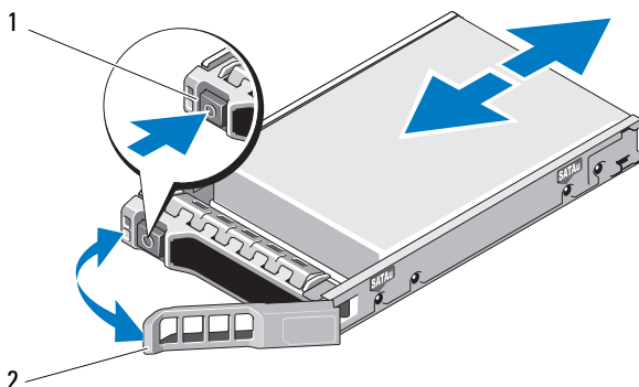
图 15-4. 卸下和安装硬盘驱动器
