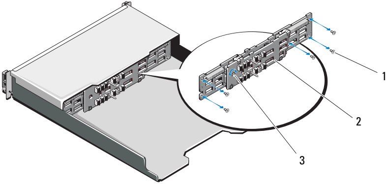
图 15-16. 卸下和安装背板 -PowerVault MD3200
