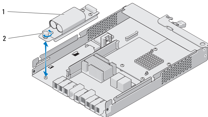
图 15-10. 卸下和安装 RAID 控制器模块备用电池装置
