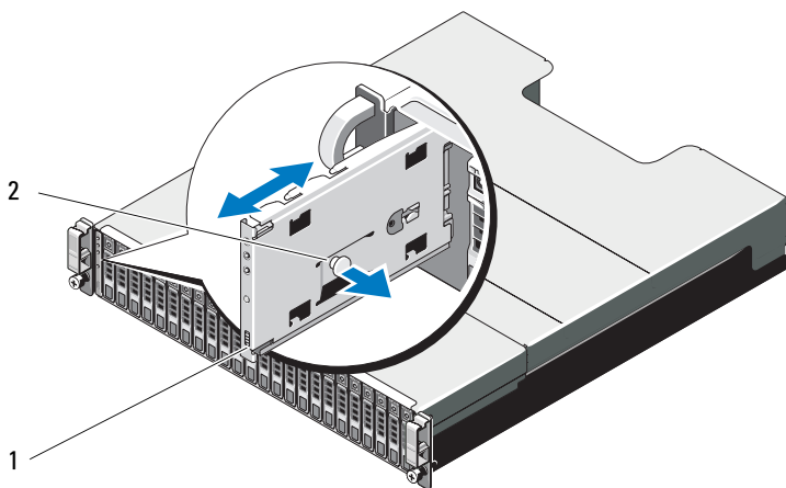
图 15-14. 卸下和安装控制面板 -PowerVault MD3220
