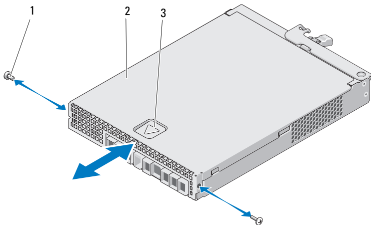
图 15-9. 打开和关闭 RAID 控制器模块
