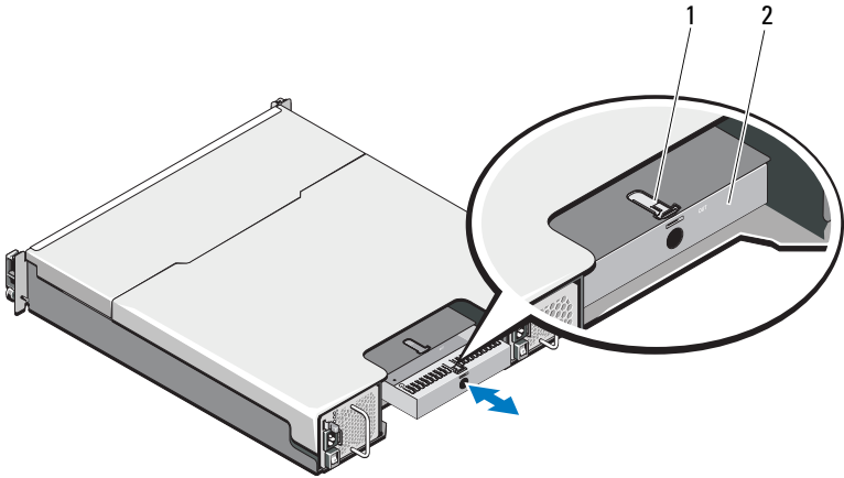
图 15-7. 卸下和安装 RAID 控制器模块挡片
