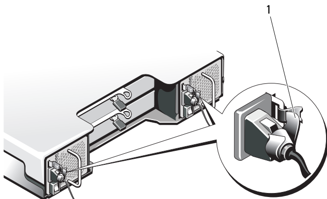
图 15-12. 固定电源电缆
