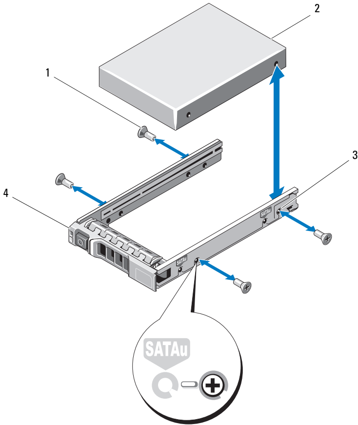
图 15-6. 卸除并安装硬盘驱动器到 2.5 英寸硬盘驱动器托盘中
