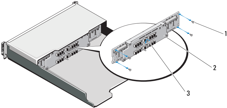
图 15-17. 卸下和安装背板 -PowerVault MD3220
